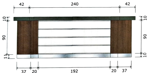
TAMPAK DEPAN Scale: 1:30
