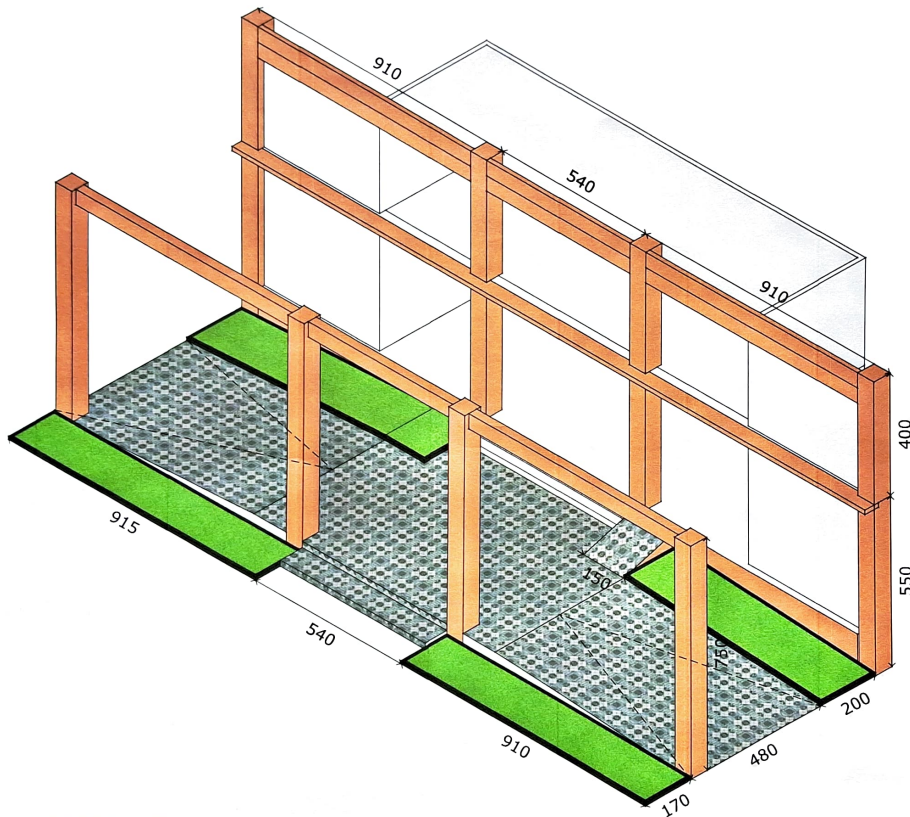
TAMPAK ISOMETRIK Scale: 1:100
