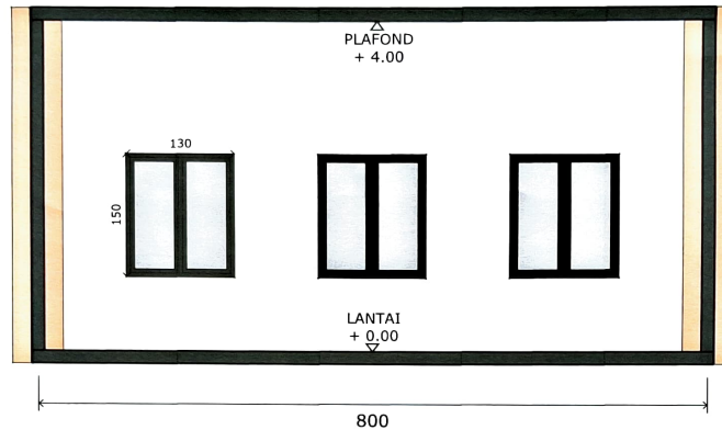
POTONGAN A-A Scale: 1:100
