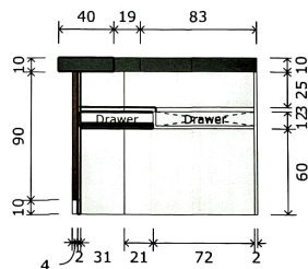
TAMPAK BELAKANG Scale: 1:30
