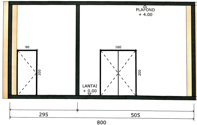
POTONGAN B-B Scale: 1:100
