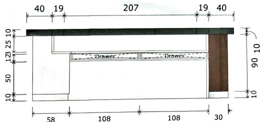
TAMPAK BELAKANG Scale: 1:30
