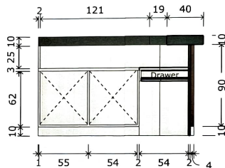
TAMPAK BELAKANG Scale: 1:30
