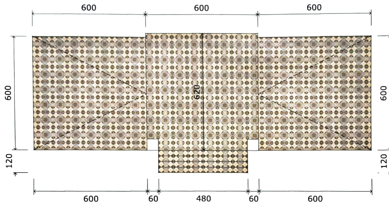
TAMPAK ATAS Scale: 1:100
