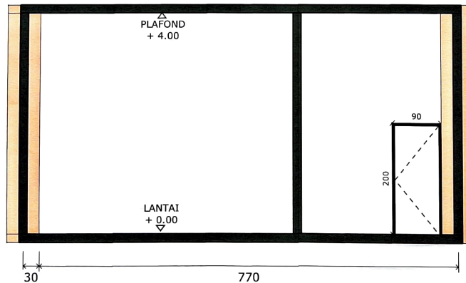
POTONGAN B-B Scale: 1:100
