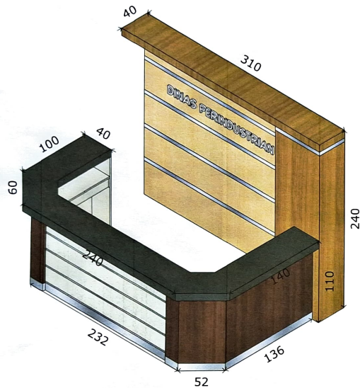
TAMPAK ISOMETRIK Scale: 1:30
