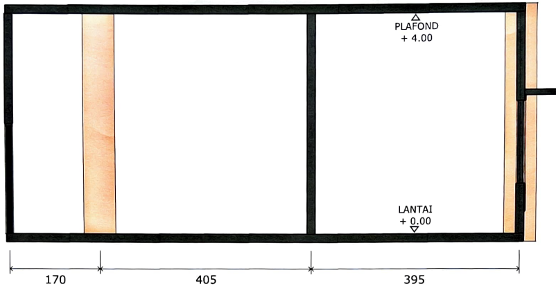
POTONGAN 1-1 Scale: 1:100
