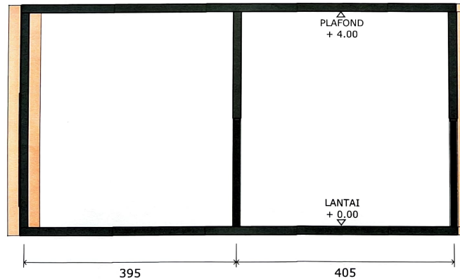
POTONGAN 2-2 Scale: 1:100
