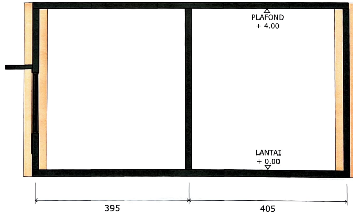
POTONGAN 2-2 Scale: 1:100
